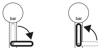
图 8：压力表截止阀关闭/打开 - 原理图
