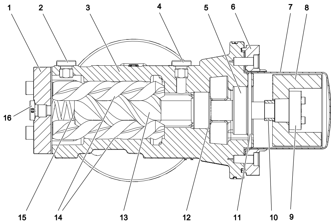
图 3: 泵结构
