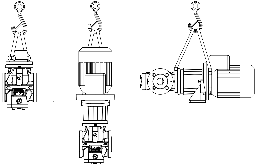
图 5: 固定起重装置 - 原理图
