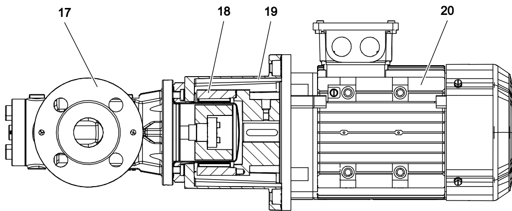
图 4: 泵组结构
