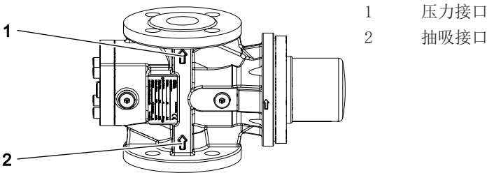
图 6：流动方向
