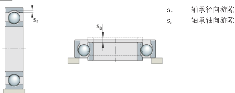
图 13: 轴承游隙
