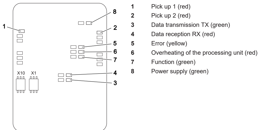
Fig. 10: Status LEDs
