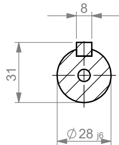
SECTION A-A (1 : 2)
