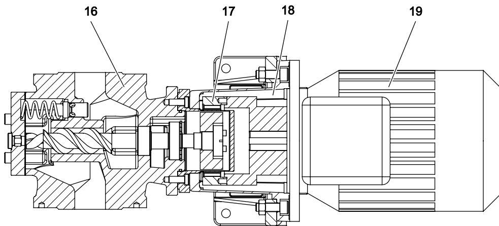
图 4: 泵组结构
