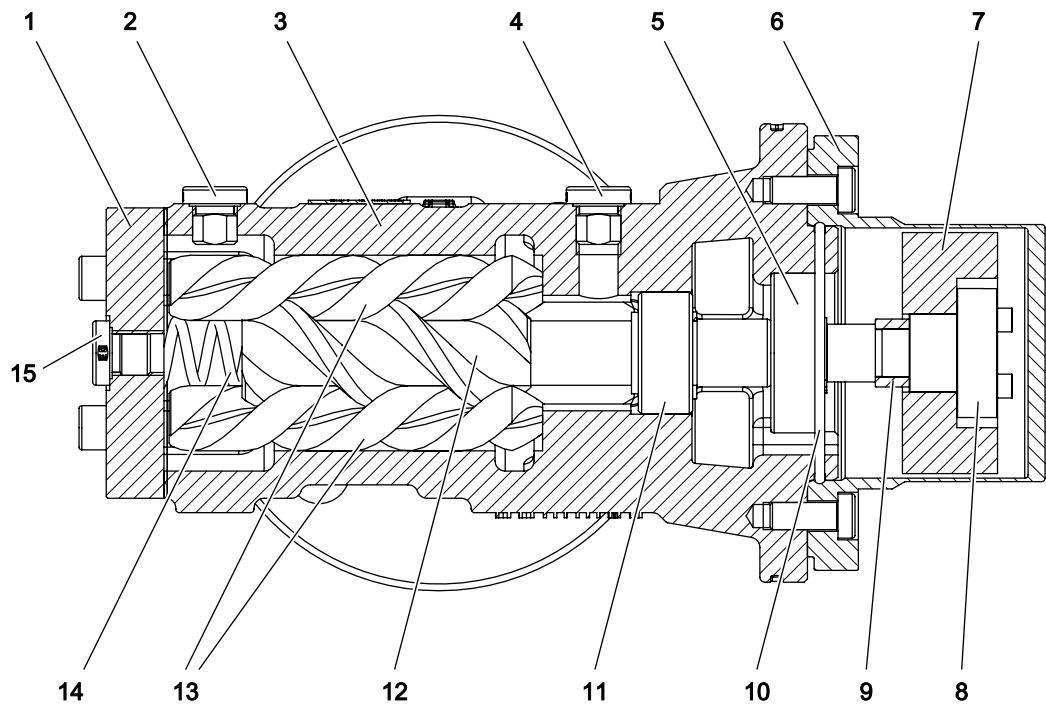
图 3: 泵结构
