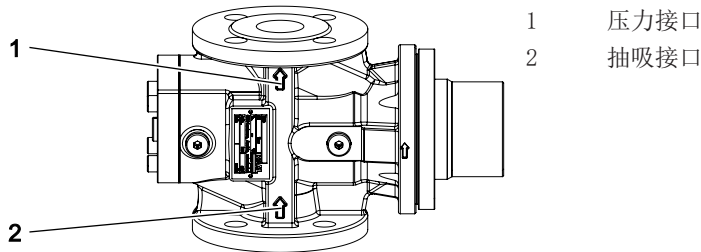
图 6：流动方向
