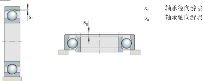
图 13: 轴承游隙
