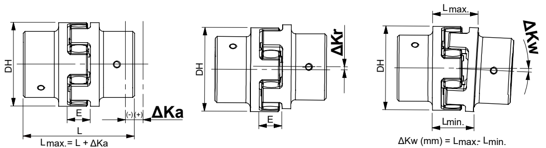
图 9：联轴器对齐测量点
