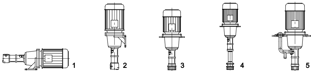
图 7: 安装方案
